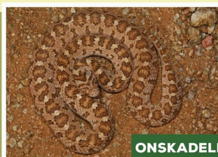
Gewone Eiervreter Daspeltis scabra
